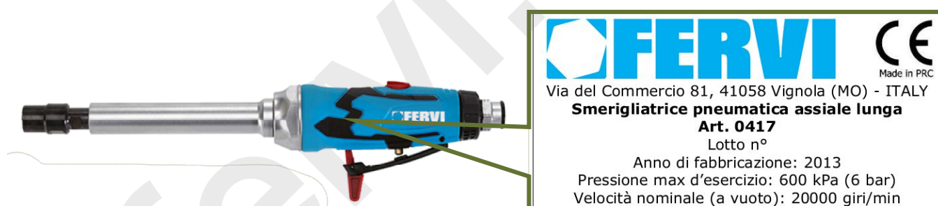
Figura 3 – Dettaglio targhetta di identificazione
